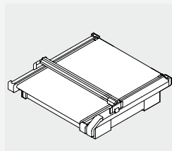
G3 2XL-3200 2740 x 3200 mm 107" x 125"
